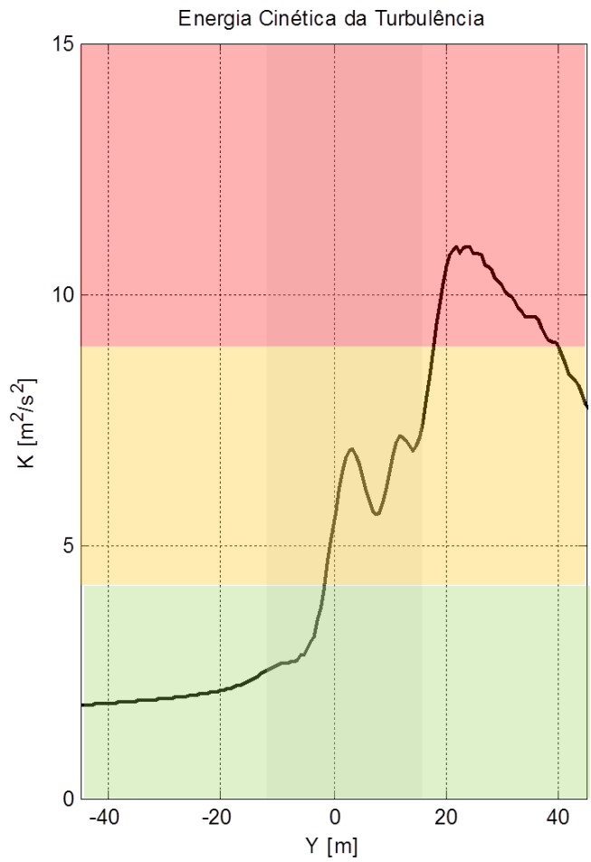
Linha de Referência, 5m acima do heliponto
